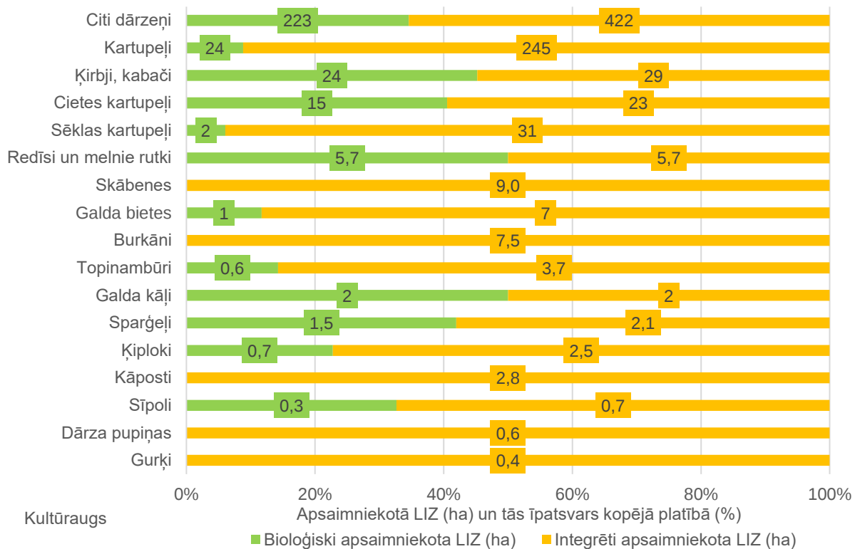
2.8. attēls. Cēsu rajona lauku partnerības teritorijā apsaimniekotā LIZ dalījumā pēc dārzeņu kultūraugiem un saimniekošanas veida 2022. gadā
